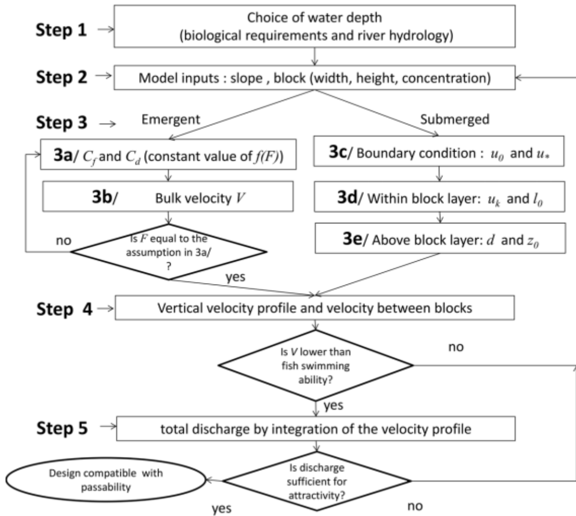
Figure 1.39: Organigramme de la méthode de calcul
